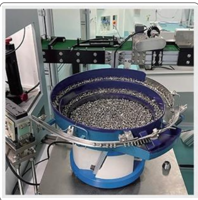
振动盘上料
