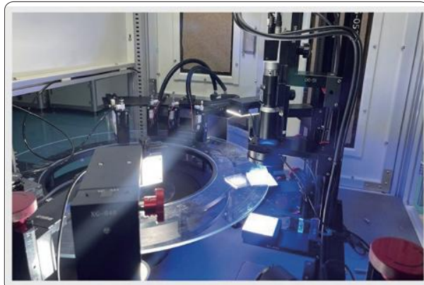
玻璃筛选盘
